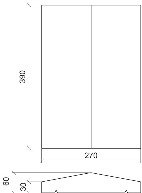
stříška průběžná
